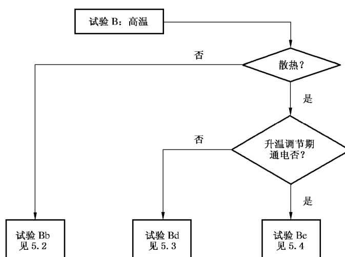
图 1 试验 B: 高温试验方框图
